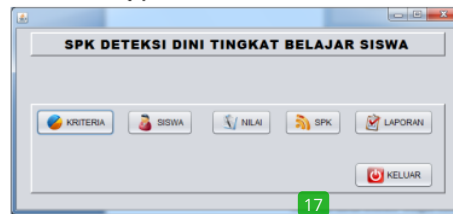
Gambar 4. Menu Utama
