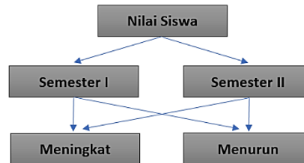
Gambar 1. Struktur Hierarki
