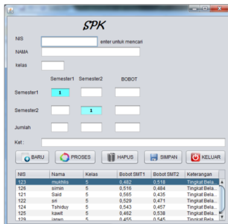
Gambar 6. Proses Keputusan
